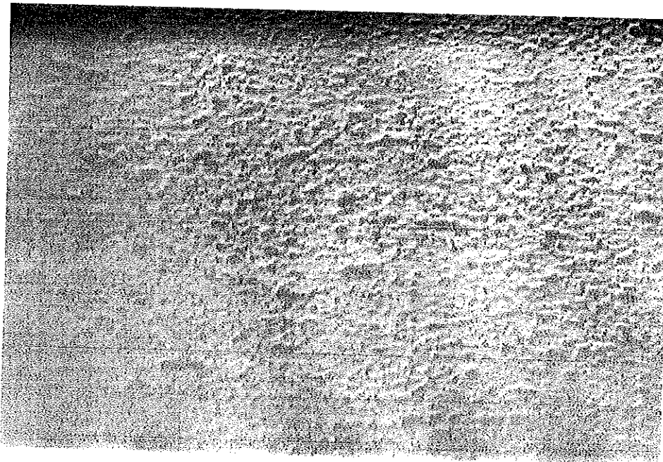
Foto 4: Roca de textura pegmática (Espigares 2016).
